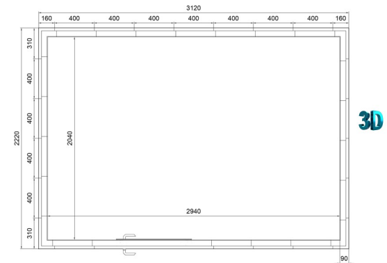
Studio - Plus - VI = 22850,00 € Int. 6.0 m2 Ext. 6.9 m2 m - 1688 kg.
