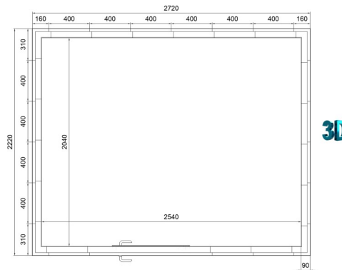
Studio - Plus - V = 19970,00 € Int. 5.2 m2 Ext. 6.0 m2 m - 1533 kg.
