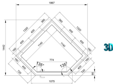
Studio - Plus - A - Multi - Angle = 7760,00 € Int. 1.2 m 2 Ext. 1.6 m 2 - 589 kg.
